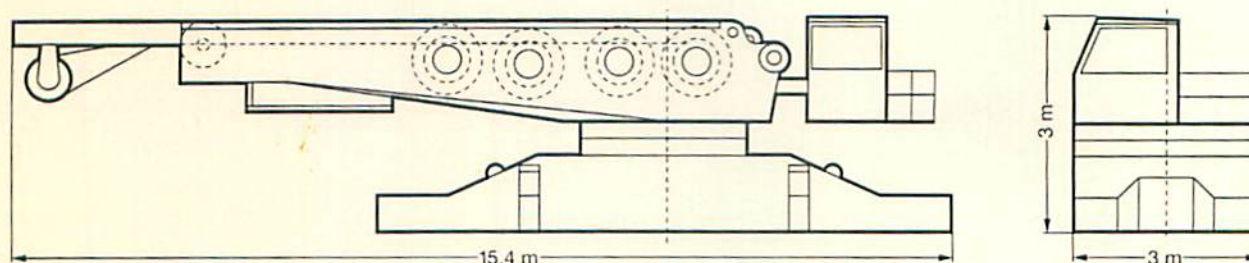
Raupenmittelteil mit Drehbühne / Crawler center frame with superstructure / Partie centrale avec partie tournante
