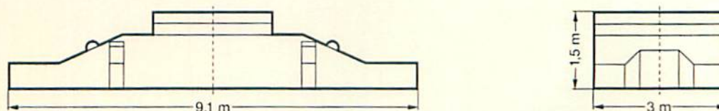
Raupenmittelteil / Crawler center frame / Partie centrale
