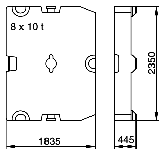
Central ballast · Zentralballast · Lest central
